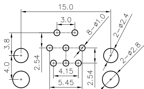
4pin A Coding
